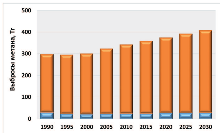
Рисунок 6.15. Оценки глобальных антропогенных выбросов метана в Мт CH 4 (оранжевым цветом) до 2030 года с выделенной долей Российской Федерации (голубым цветом). Диаграмма составлена по данным Агентства по защите окружающей среды США (EPA, 2012)
