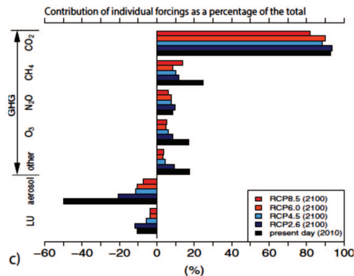
Рисунок 8.2. Вклады различных парниковых веществ – CO 2 , CH 4 , N 2 O, O 3 , других парниковых газов и аэрозолей – в суммарное радиационное воздействие (с начала индустриальной эры) в 2100 г. в условиях четырех сценариев RCP и в 2010 г.: верхняя панель – абсолютные величины, нижняя панель – % (Meinshausen, 2011; Collins et al, 2013, p. 1046)
