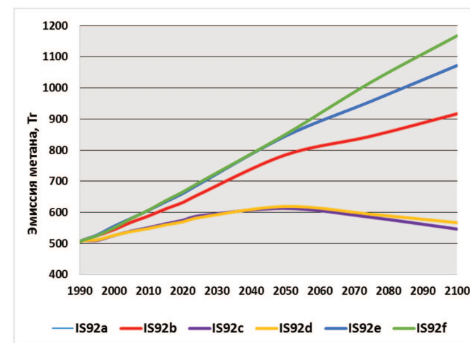
Рисунок 6.17. Глобальные антропогенные выбросы метана (Мт CH 4 ) до 2100 года, построенные на базе сценариев семейства моделей IS92. Составлено по данным работ (Leggett J. et al, 1992; Pepper et al, 1992)
