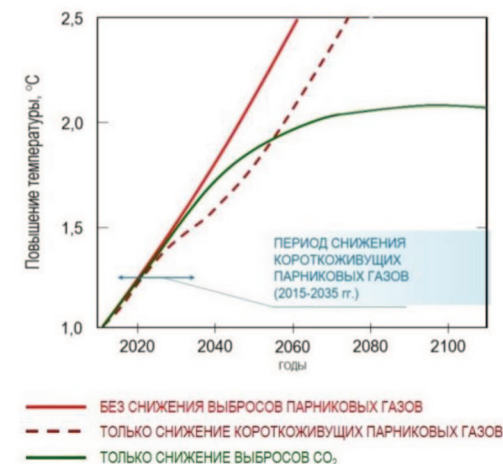
Рисунок 13.3. Вклад \text{CO}_2 и короткоживущих парниковых газов в удержание глобальной температуры
