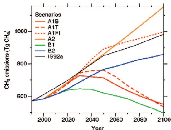
Рисунок 6.18. Глобальные антропогенные выбросы метана (Мт \text{CH}_4 ) в 1990–2100, соответствующие сценариям SRES – Специального доклада МГЭИК о сценариях выбросов (IPCC, 2000)
