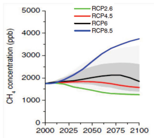
Рисунок 6.21. Ход глобальной концентрации CH 4 (ppb) в XXI веке в условиях сценариев RCP (Clarke et al, 2010; van Vuuren et al, 2011)
