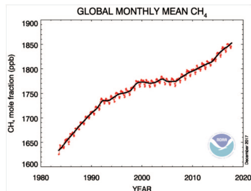
Рисунок 6.11. Изменение среднемесячных глобальных значений концентрации \text{CH}_4 в приповерхностном слое (Dlugokencky, NOAA/ESRL ( www.esrl.noaa.gov/gmd/ccgg/trends_ch4/ ; Nisbet et al., 2016)
