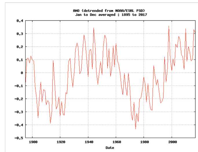
Рисунок 9.2. График температурных изменений в вечномёрзлотных областях Гренландии (1900 – 2017 гг.). Источник: [99] ( http://sciencenordic.com/greenland%E2%80%99s-recent-temperature-drop-does-not-disprove-global-warming )
