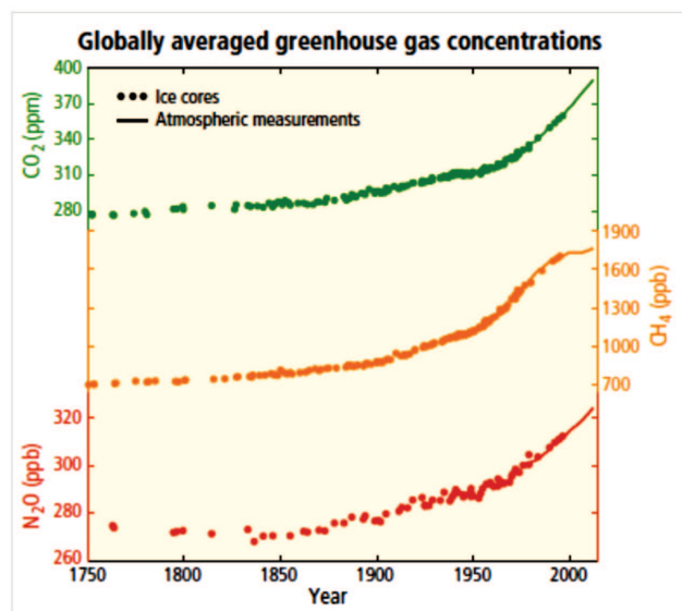
Рисунок 6.14. Глобальные концентрации углекислого газа \text{CO}_2 (зеленый цвет), метана \text{CH}_4 (оранжевый цвет) и закиси азота \text{N}_2\text{O} (красный цвет) – данные реконструкции по ледовым кернам и результаты инструментальных измерений (IPCC, 2014)
