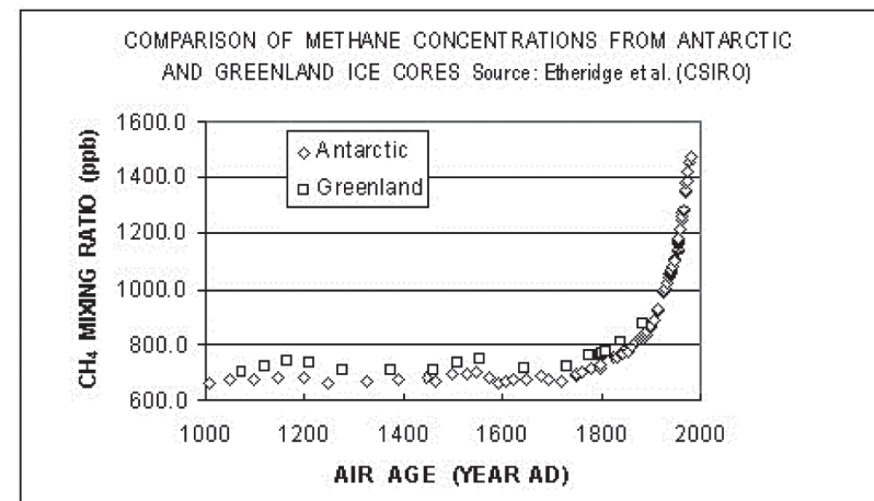
Рисунок 3.3. Ход концентрации метана с 1000 г. в Антарктиде и Гренландии (Etheridge et al, 2002)
