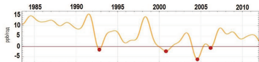
Рисунок 13.2. Динамика роста/снижения концентрации метана в атмосфере
