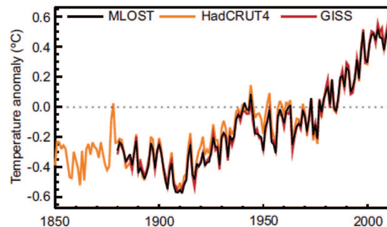
Рисунок 6.10. Ход средней глобальной температуры (изображены три различных ряда данных наблюдений – MLOST, HadCRUT4 и GISS) в приповерхностном слое в 1850-2012 гг. по отношению к среднему значения за 1961-1990 гг. (IPCC, 2013, p. 193)
