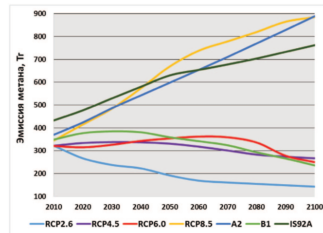
Рисунок 6.22. Сопоставление глобальных антропогенных выбросов метана в 2010–2100 гг. в условиях сценариев различных семейств; график составлен по данным (IPCC, 2013)
