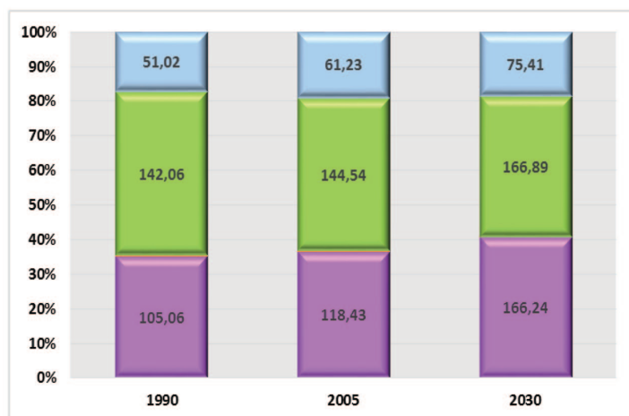
Рисунок 6.16. Глобальные антропогенные выбросы метана в Мт CH 4 в 1990, 2005 и 2030 годах с детализацией по основным секторам экономики – источникам эмиссии метана. Вклады показаны различными цветами: энергетики (голубым), сельского хозяйства (зеленым), отходов (сиреневым). Диаграмма составлена по данным Агентства по защите окружающей среды США (EPA, 2012)
